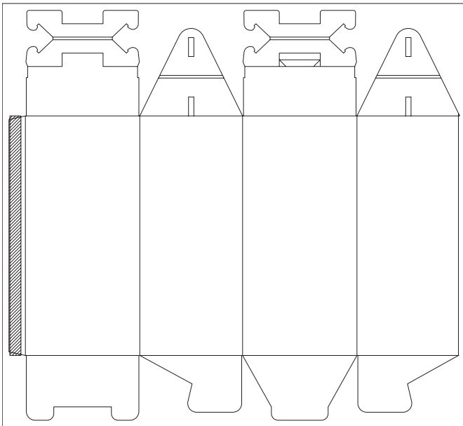
Caisse à rabats fond emboîté avec poignée 254 x 228 x 530 mm ondulation blindée
